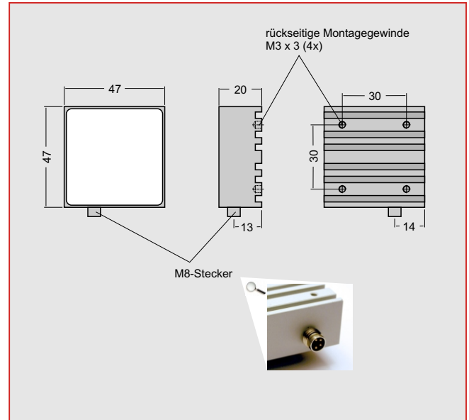
TOP-LIGHT-40 Gehäuse mit integrierten Kühlrippen
