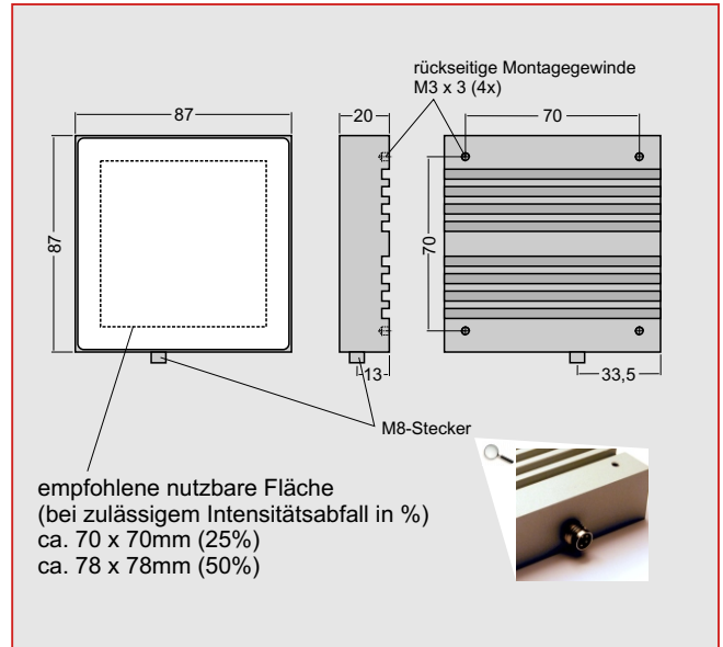
HI-LIGHT-80 Gehäuse mit integrierten Kühlrippen
